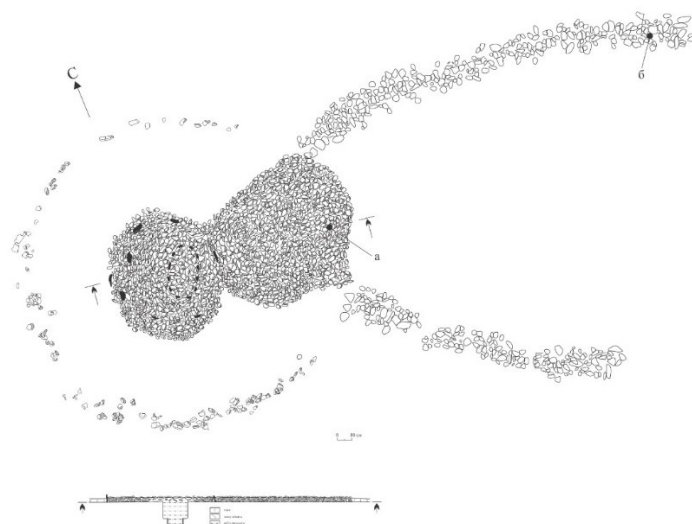
Сурет 2 – Сарытау «мұртты» обасының жоспары мен қимасы [Fig. 2 – Plan and Section of the Sarytau Barrow with «Moustache»]
