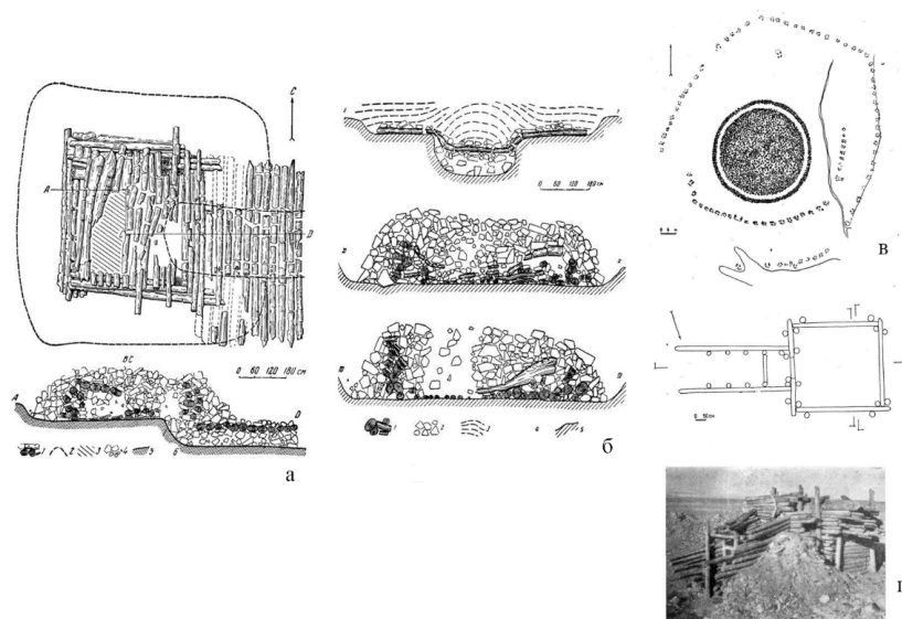
Рис. 4 – Деревянное сооружение курганов Чиликты V и Бешатыра [по 35, Табл. III–IV и 36, Рис. 3, 15-16.]
